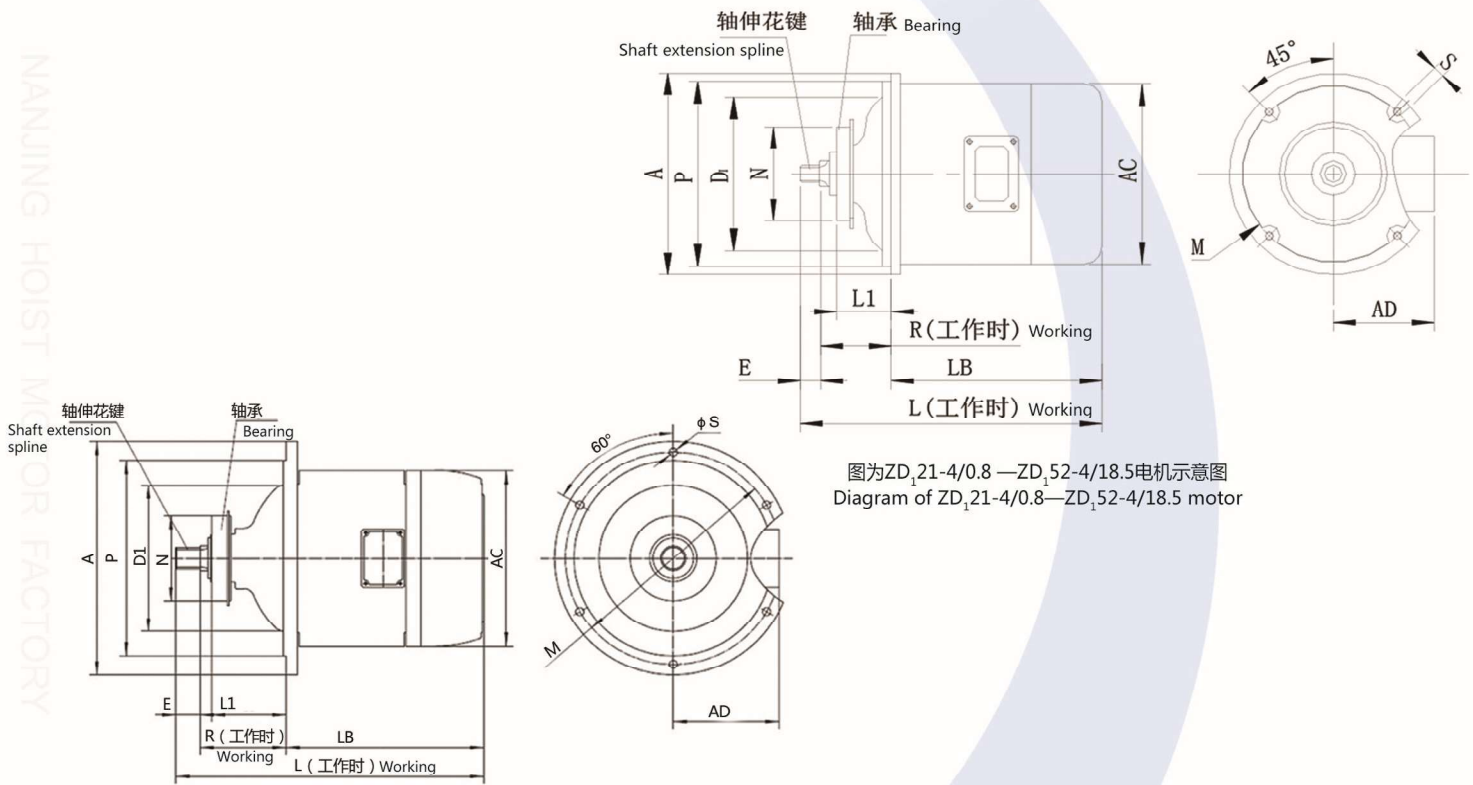
图 2 为ZD 1 52-4/18.5D—ZDX62-6/18.5电机示意图 Diagram of ZD 1 52-4/18.5D—ZDX62-6/18.5 motor
